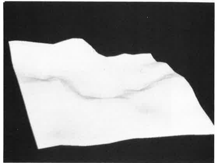
(a) DEM only
